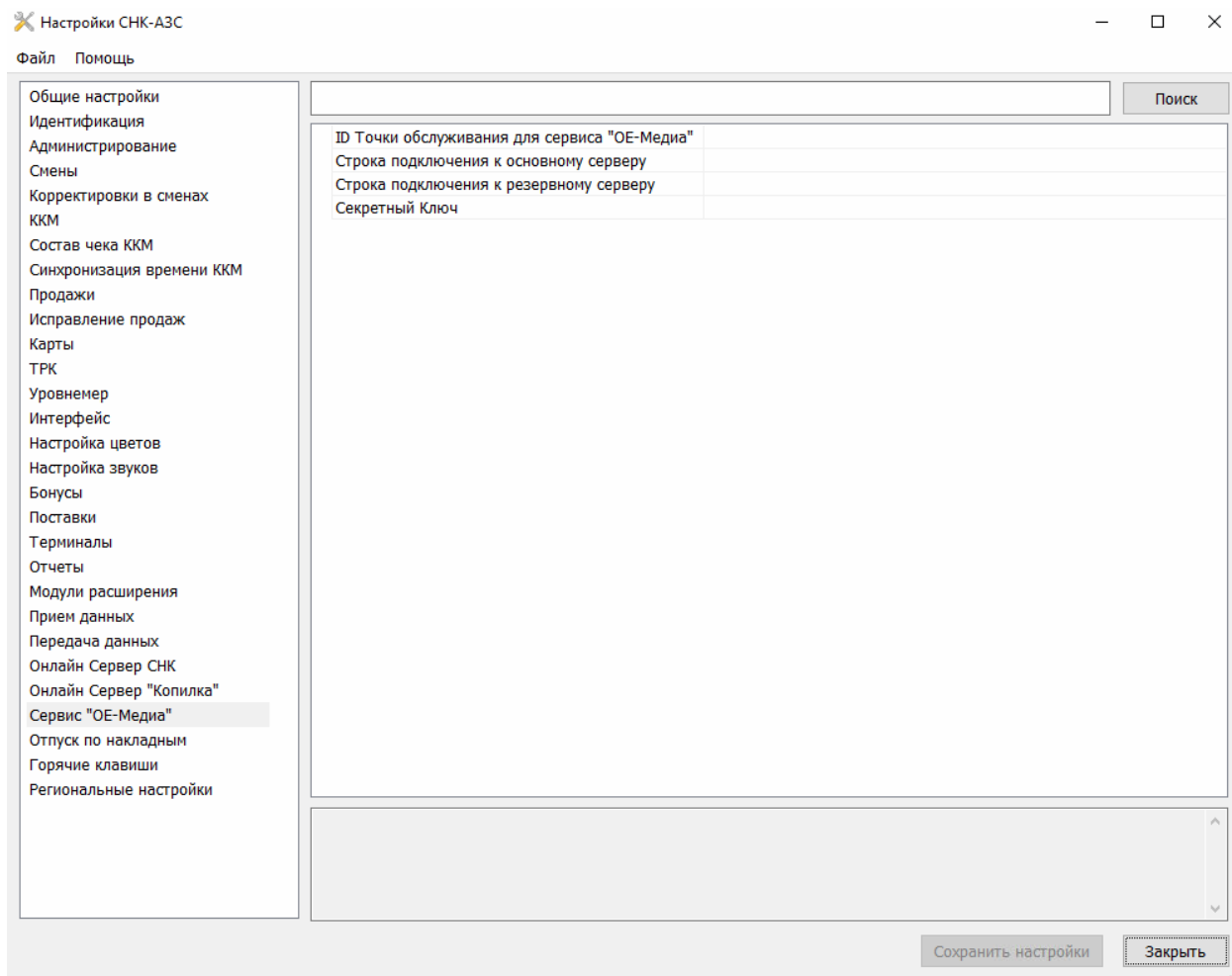
Рисунок 1. – Настройка подключения
