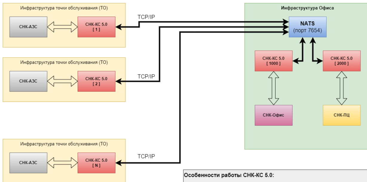
Структурная схема коммуникационного пакета СНК-КС 5.0
